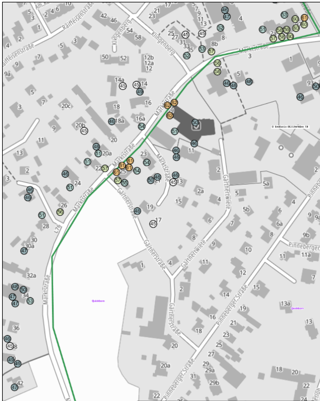
Abbildung 10: Fassadenpunkte L_{\text{Night}} Marktstraße, L76
